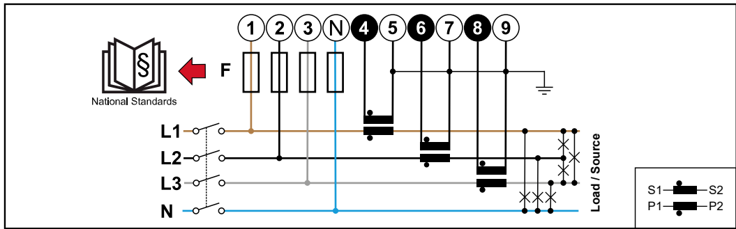
3 Phasen, 4 Leiter (CT-Anschluss)
