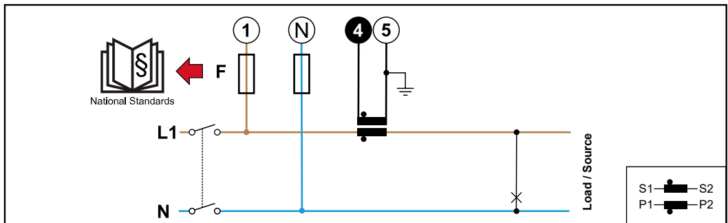
1 Phase, 2 Leiter (CT-Anschluss)
