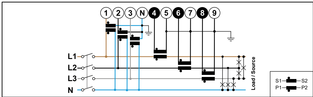
3 Phasen, 4 Leiter (VT/CT-Anschluss)
