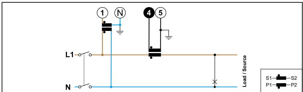
1 Phase, 2 Leiter (VT/CT-Anschluss)
